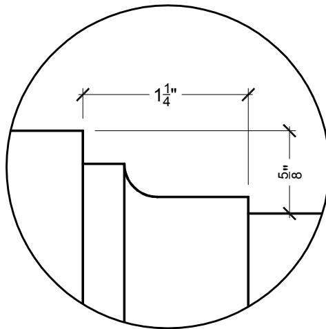
1 DETAIL SCALE: 1" = 1"
