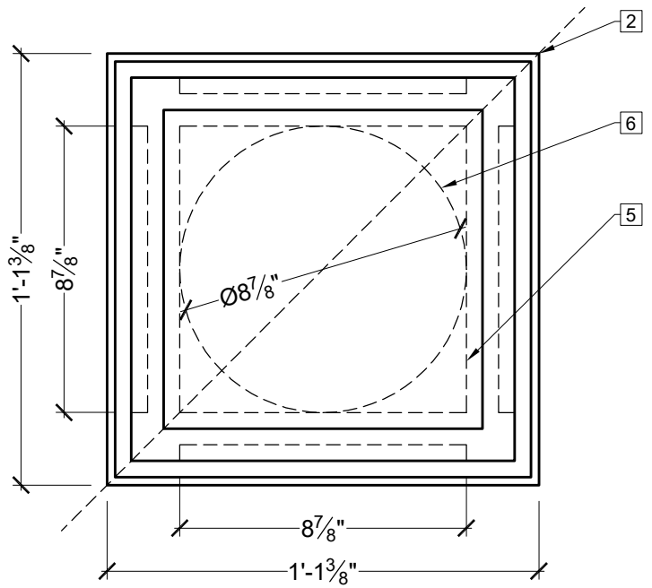
A TOP VIEW SCALE: \frac{3}{16}'' = 1''
