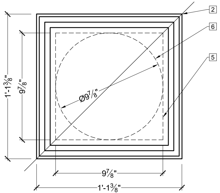
(A) TOP VIEW SCALE: \frac{5}{16}'' = 1''
