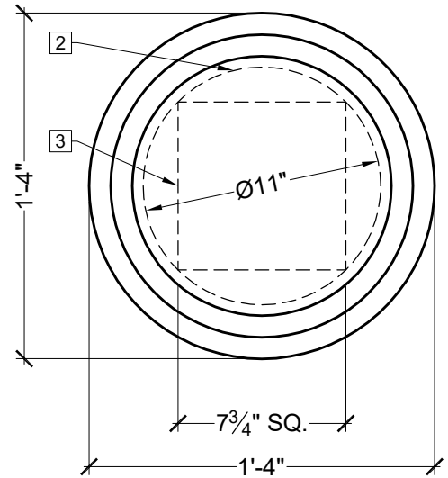
TOP VIEW SCALE: \frac{1}{8}'' = 1''
