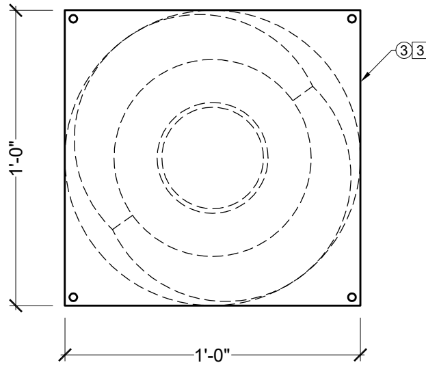
TOP VIEW SCALE: \frac{3}{16}'' = 1''
