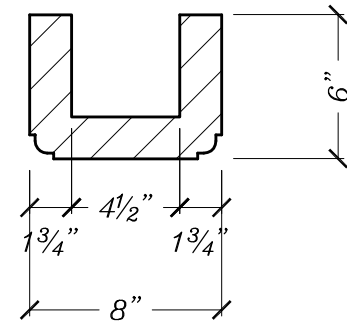
END VIEW SCALE: 1/8" = 1"
