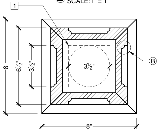
B DETAIL A SCALE: 1" = 1"
